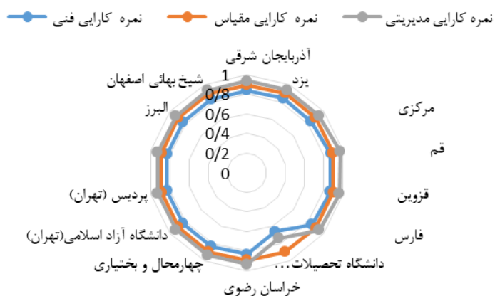
شکل شماره ۶: نمودار مقادیر کارایی پارک‌ها در شهرهای صنعتی
